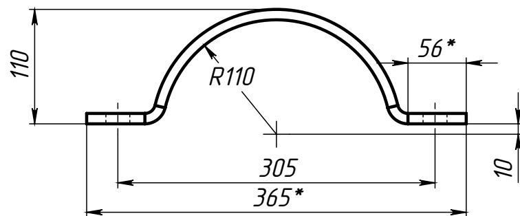
Поз.4 (Полухомут)
